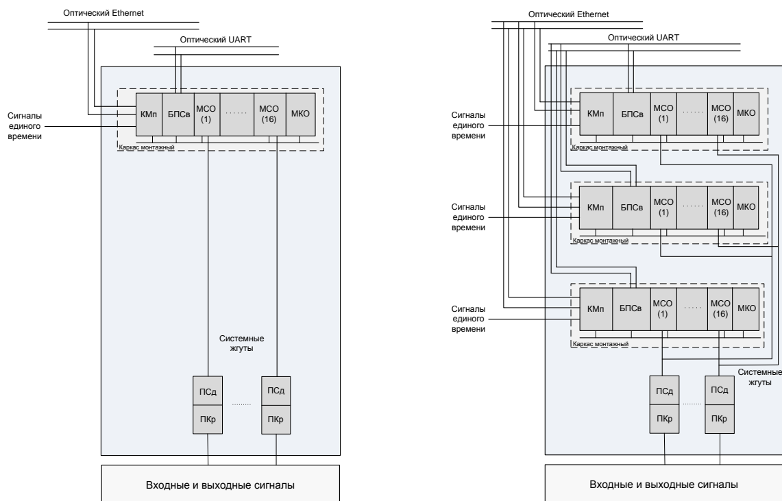
Структурные схемы МСКУ-3 без резервирования и с трехкратным резервированием
